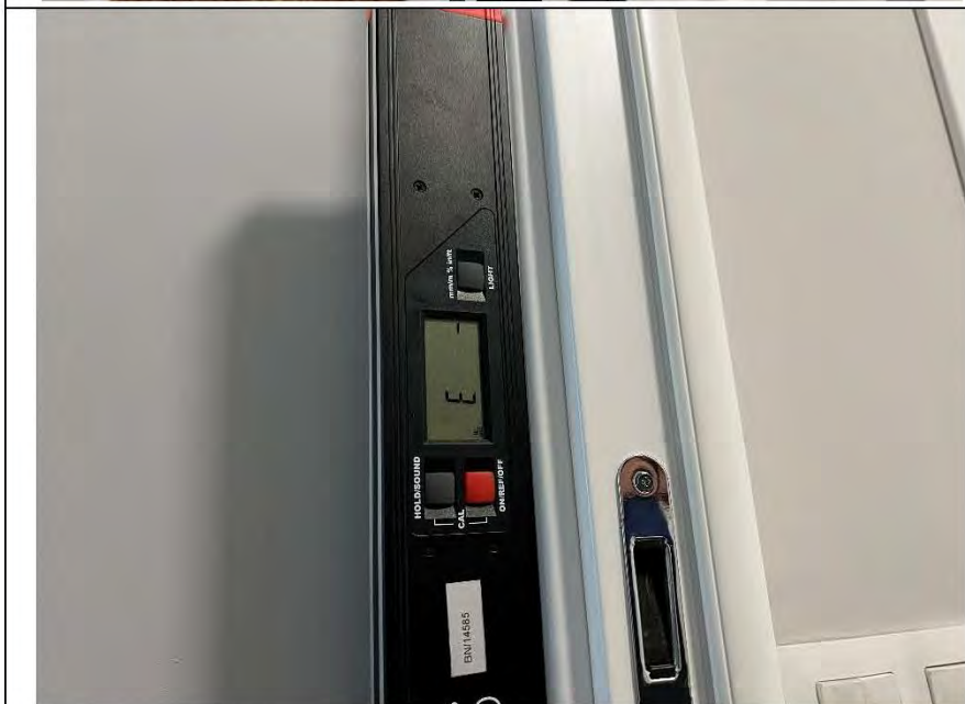
Фото №42. Отклонение наличников дверного блока в кухне равно 3 мм.
