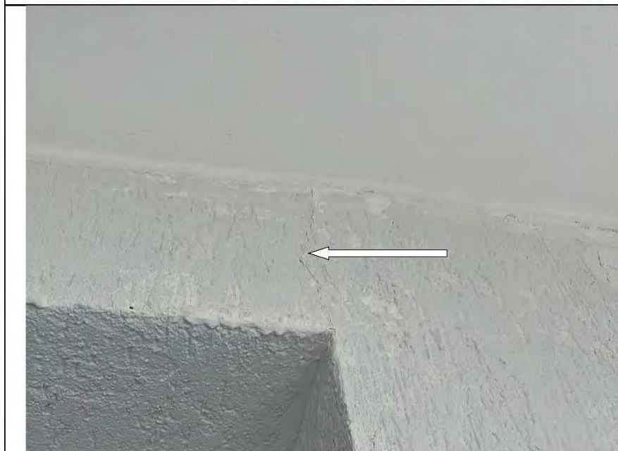
Фото №11. Трещины на окрашенных стенах на лоджии.
